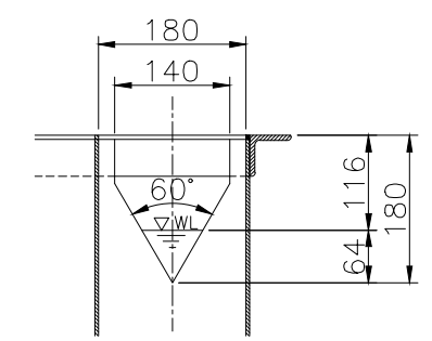
A-A矢视图 S=1/10
